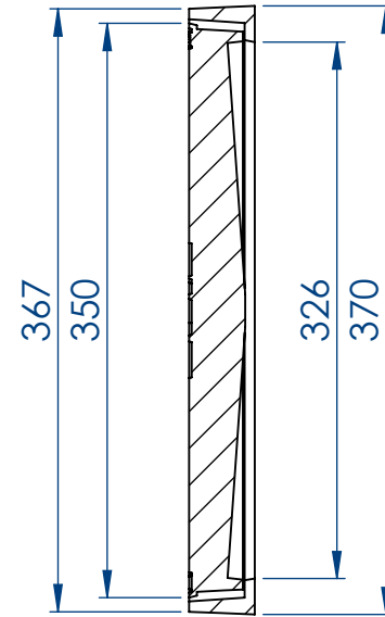
KESIT B-B
